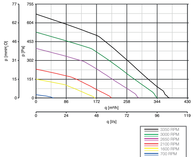
VORT PROMETEO PLUS HR 400 WYDAJNOŚĆ/ CIŚNIENIE STATYCZNE
